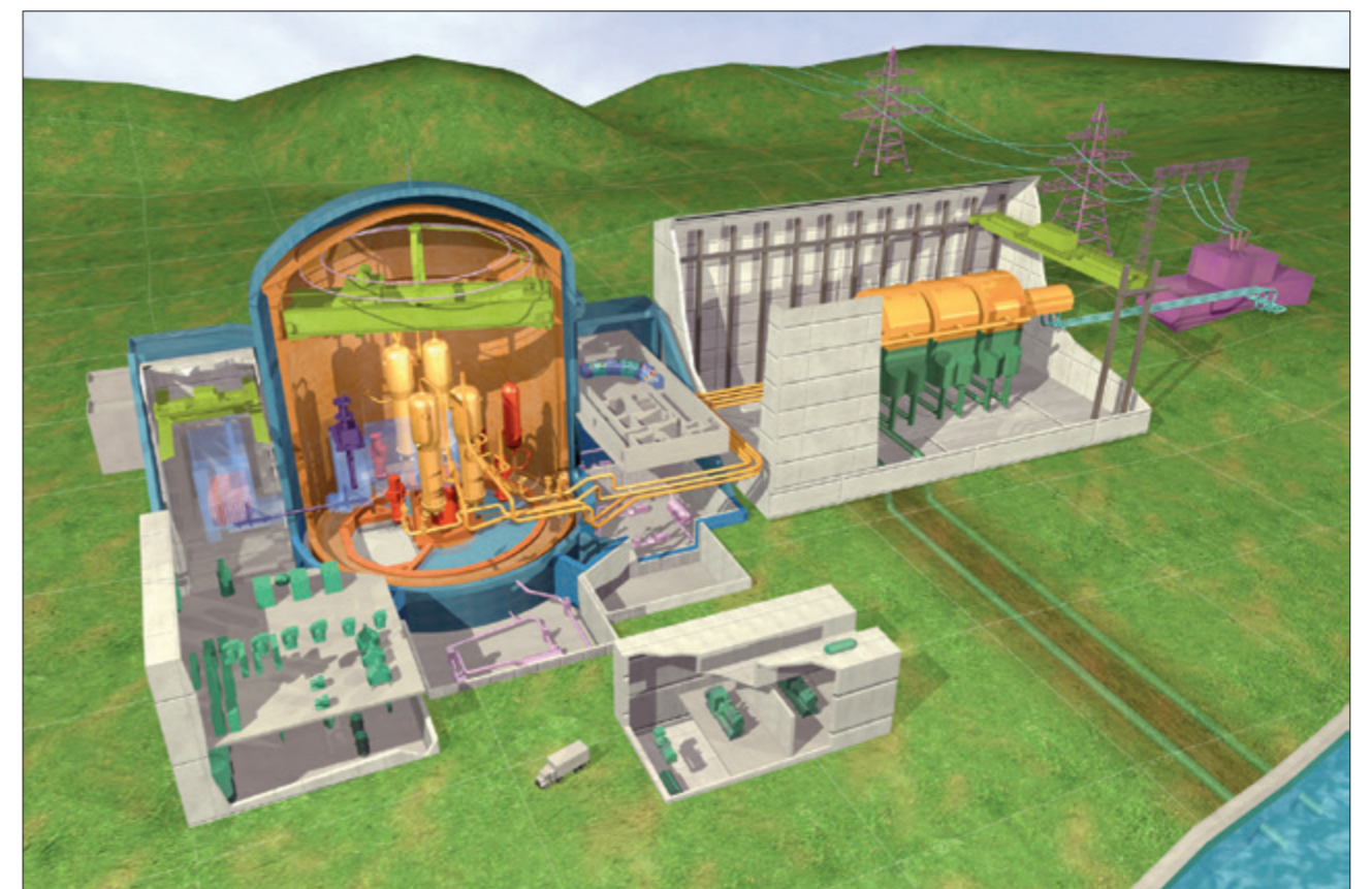
Schnitt durch den Aufbau des im Bau befindlichen EPR Reaktors in Olkiluoto, Finnland. Dabei handelt es sich um einen Kernspaltungsreaktor der III. Generation. (© Framatome GmbH)
