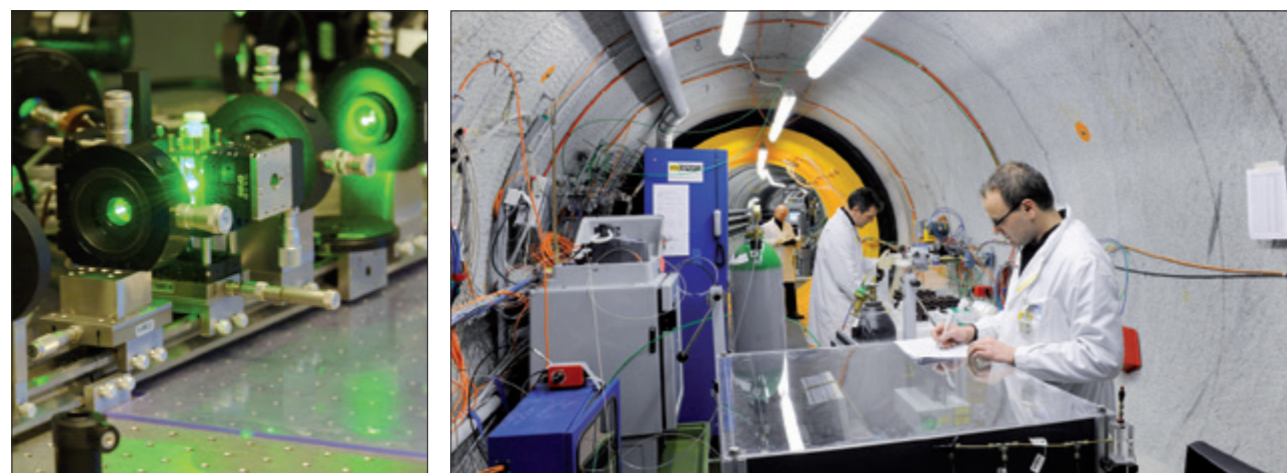
Links: Aufbau zur Aufklärung der chemischen Form gelöster Actinidionen mittels Laserspektroskopie (© KIT, Coerten); rechts: Experimente zur Radionuklidmigration im Grimsel Felslabor, Schweiz (© COMET, Photoshopping, GmbH, Weisslingen)
