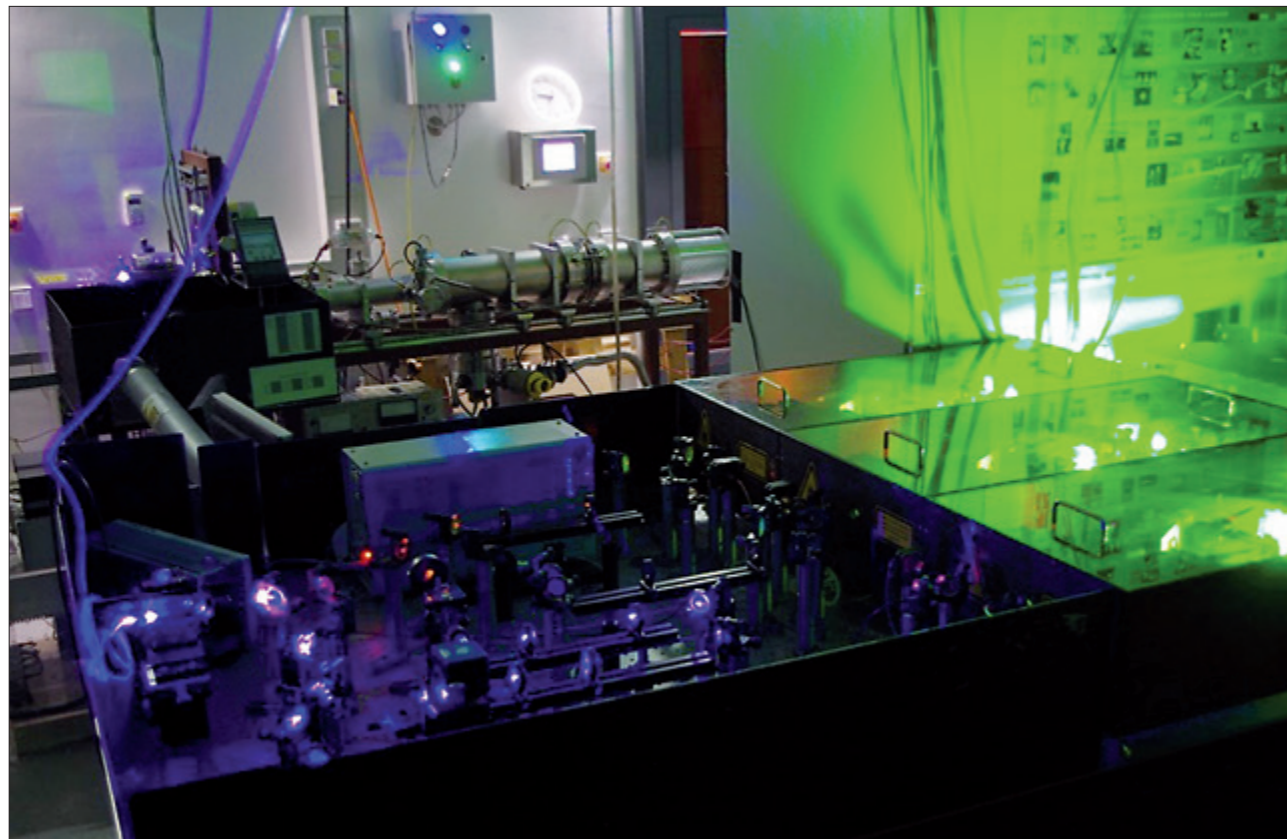
Das Foto zeigt im Vordergrund die Laserapparatur für die Resonanzionisations-Massenspektrometrie (RIMS), die am Institut für Kernchemie der Universität Mainz zum Ultraspurenachweis von Plutonium, Neptunium und Technetium eingesetzt wird. Mit dem von einem Nd:YAG-Laser erzeugten grünen Laserlicht werden drei Ti:Saphir-Laser gepumpt. Das blaue Laserlicht entsteht durch Frequenzverdopplung des von einem der Ti:Saphir-Laser abgegebenen fundamentalen Laserlichtes. Im Hintergrund ist das Flugzeit-Massenspektrometer (TOF-MS) zum Nachweis der durch die Laserstrahlung selektiv ionisierten Radioisotope zu sehen. © Nils Stöbener, Institut für Kernchemie, Universität Mainz
