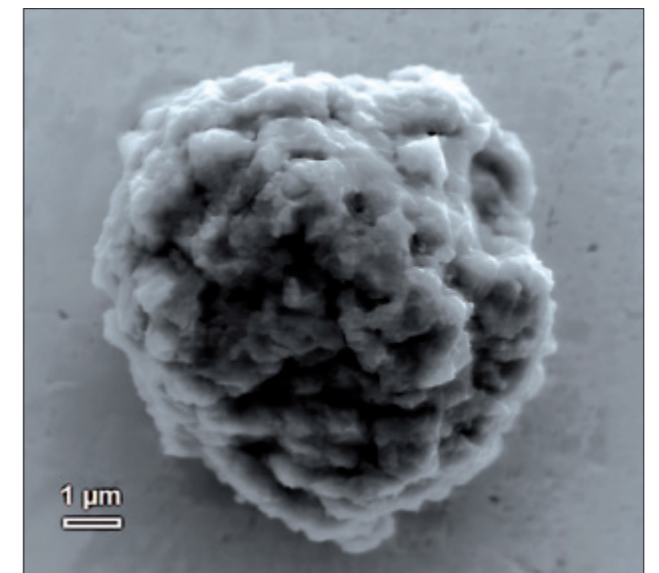
Sternenstaub von Roten Riesen – Siliziumkarbid-Korn aus dem Meteoriten Murchison. (© J. Huth, S. Merchel, MPI Mainz)
